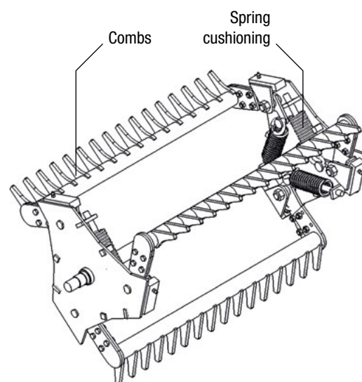
Rotor MYMESIA
