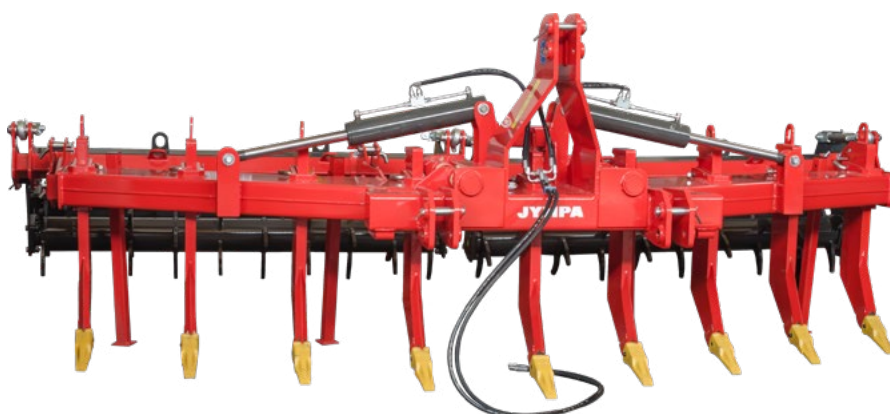
Modèle ANTARES 9-SR50-PC avec socs en acier moulé et rouleau double Ø 520 mm
