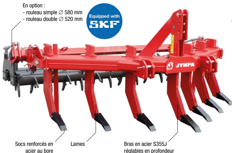
Modèle ANTARES-7 avec rouleau double Ø 520 mm
