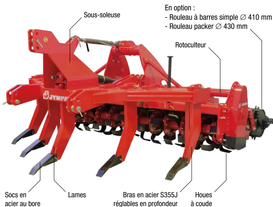
Modèle DUPLA-3000-R avec rouleau packer Ø 430 mm
