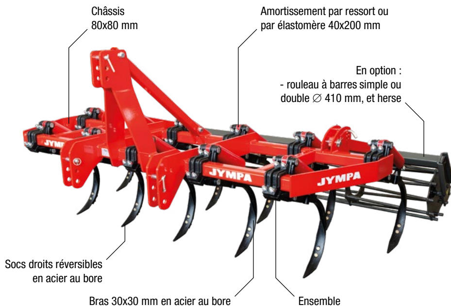
Modèle OSIRIS-11-2F avec rouleau à barres simple Ø 410 mm
