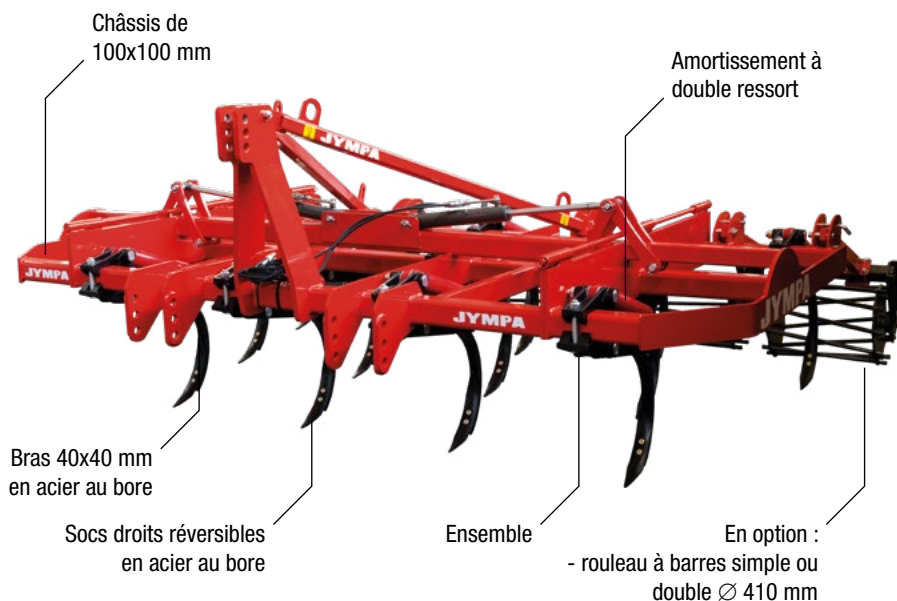
Modèle DAGON-13-3F-PL avec rouleau à barres simple Ø 410 mm
