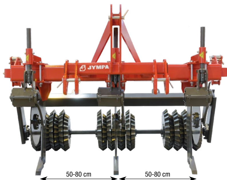
Modèle ALASIA-3-AR avec rouleau étoile Ø 500 mm et avec distance entre bras réglable mécaniquement
