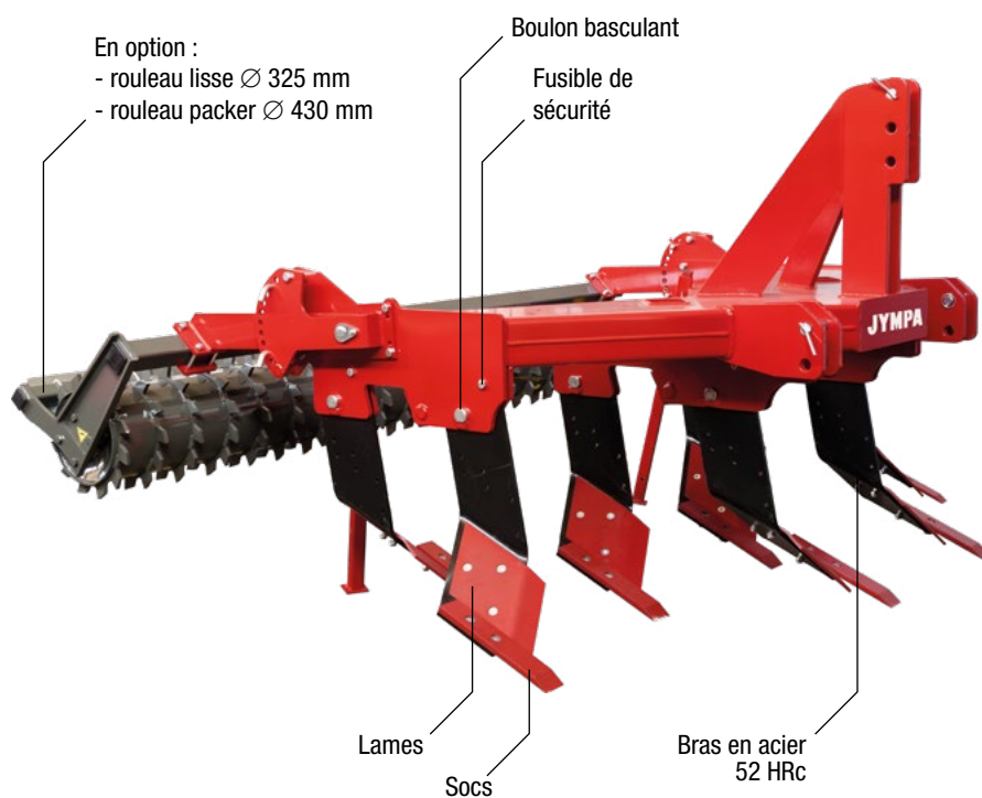
Modèle MINTAKA-4 avec rouleau packer Ø 430 mm
