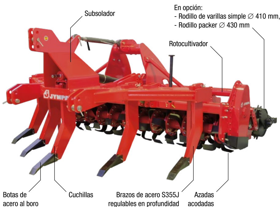
Modelo DUPLA-3000-R con rodillo packer Ø 430 mm
