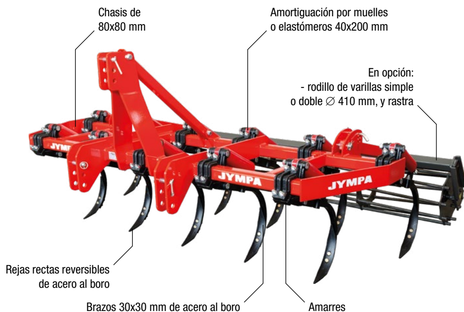
Modelo OSIRIS-11-2F con rodillo de varillas simple Ø 410 mm
