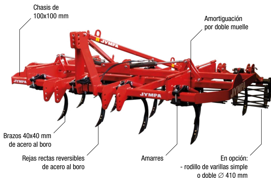
Modelo DAGON-13-3F-PL con rodillo de varillas simple Ø 410 mm
