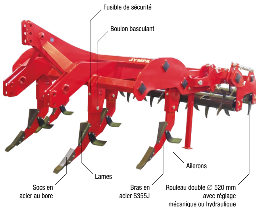
Modèle SIRIUS-5R avec rouleau double Ø 520 mm avec réglage mécanique
