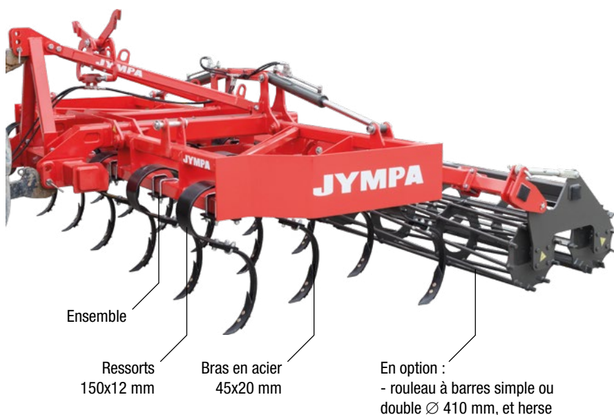
Modèle NEPER-18-3F-PC avec rouleau à barres double Ø 410 mm
