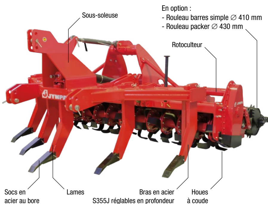
Modèle DUPLA-3000-R avec rouleau barres simple Ø 410 mm
