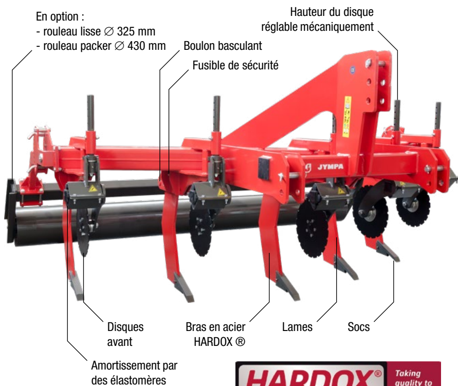
Modèle ALASIA-5 avec rouleau lisse Ø 325 mm
